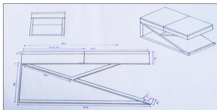
Rajah 7: Rekaan akhir meja kopi moden pelbagai guna
