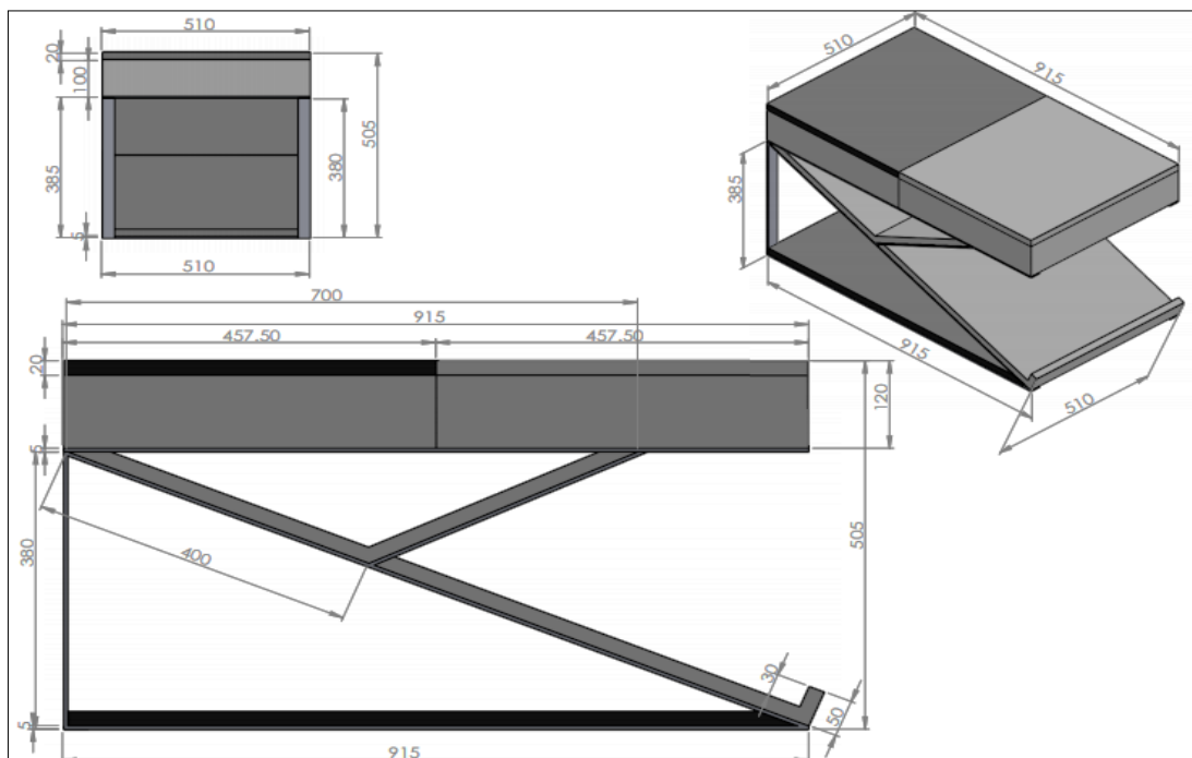
Rajah 9: Lukisan teknikal meja kopi moden pelbagai guna berinspirasikan Palmanova, Itali
